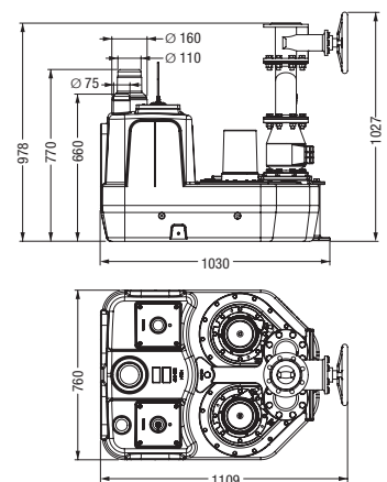
На иллюстрации исполнение Duo с чугунной задвижкой
