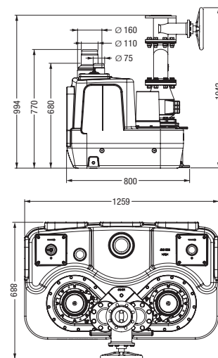
На иллюстрации исполнение Duo с чугунной задвижкой
